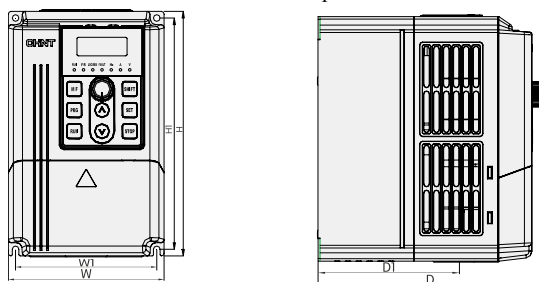
Рис. 1.3 Внешний вид преобразователя частоты (NVF2G-0.4/TD2 ~ 1.5/TD2 и NVF2G-0.75/TS4 ~ 1/PS4)
