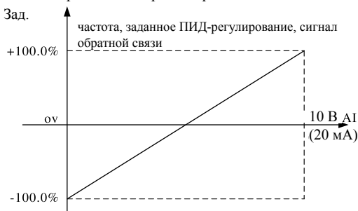
Рис. 6.12 Взаимосвязь между АИ и соответствующей настройкой
