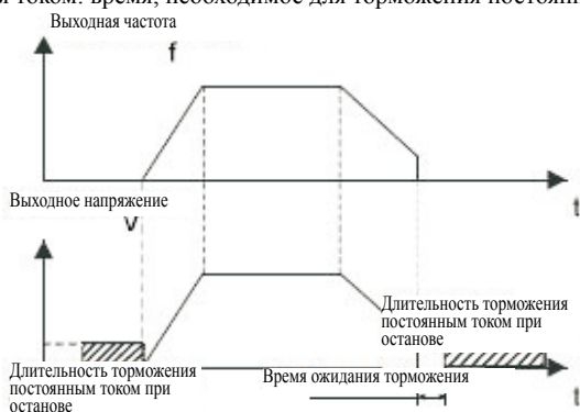
Рис. 6.3 Диаграмма торможения постоянным током
