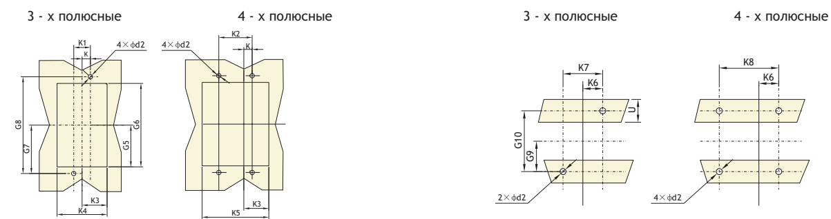
Разметка монтажной панели
