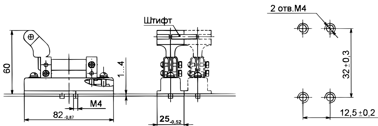
Разъединитель Р-25-1111 Масса 0,08 кг
