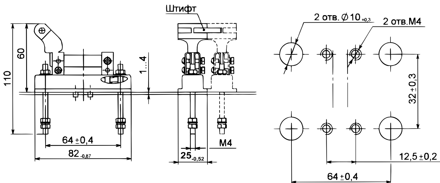
Разъединитель Р-25-1121 Масса 0,102 кг
