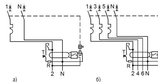
Рисунок Г.1 - Принципиальные электрические схемы АВДТ а) двухполюсного; б) четырехполюсного Т – устройство эксплуатационного контроля (кнопка «ТЕСТ») R – токоограничивающее сопротивление
