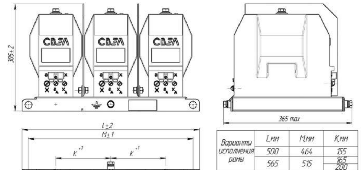
Рис.2 Клеммник трансформатора ЗНОЛ(П)-СВЭЛ-6(10)
